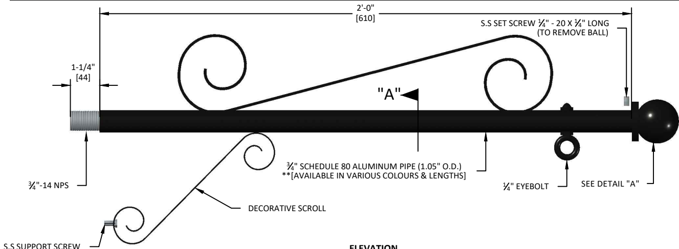
ELEVATION
