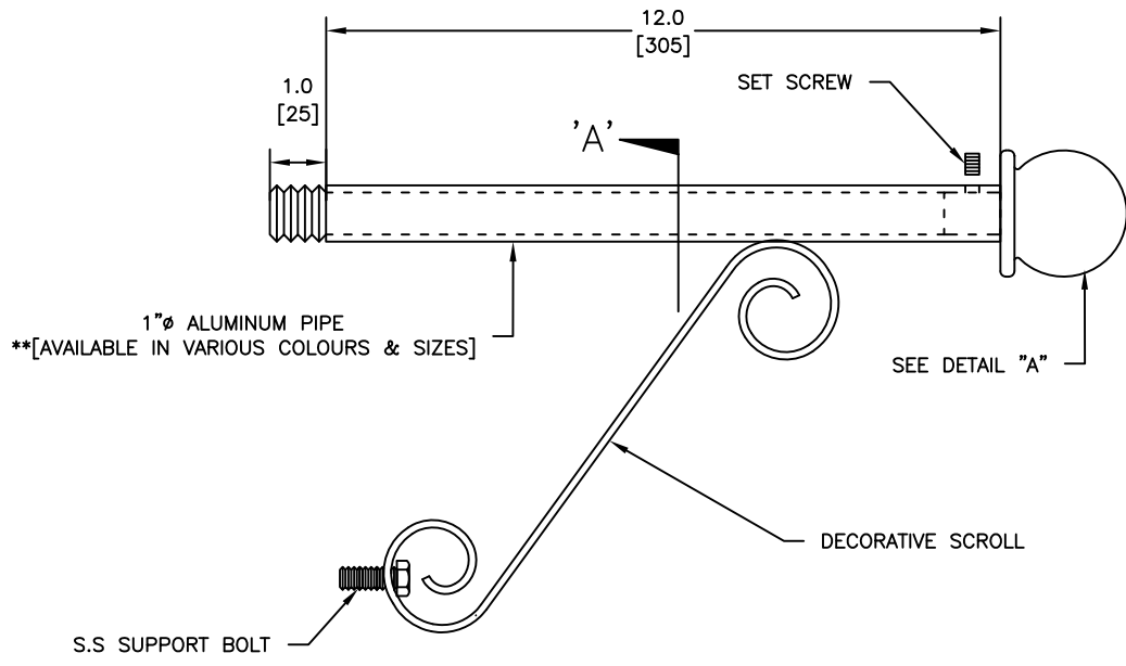
ELEVATION
