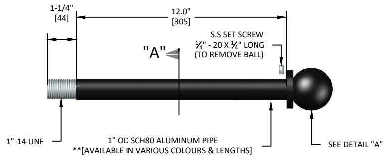
ELEVATION
