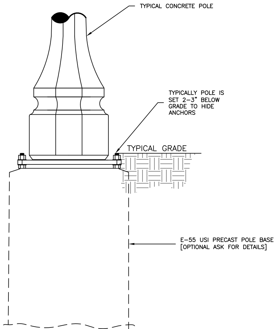
ELEVATION
