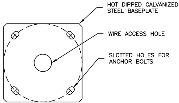
BASEPLATE
