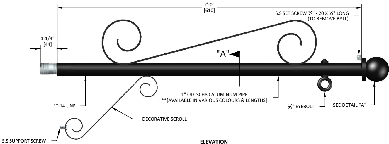
ELEVATION
