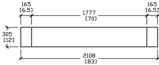
END ELEVATION
