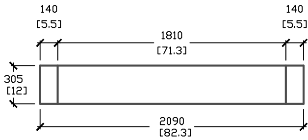
END ELEVATION
